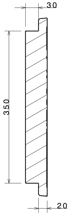
Section view B-B Scale: 1:5
